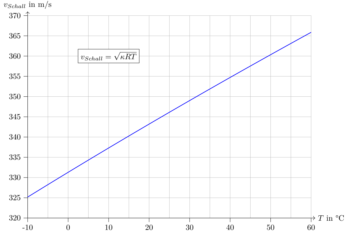
Figure 7.2.: Ausbreitungsgeschwindigkeit von Schall in Luft
