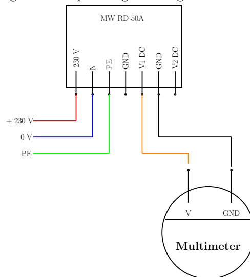
Figure 9.3.: Spannungsmessung des Netzteils
