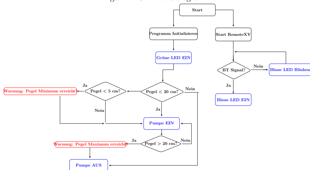
Figure 14.5.: Ablaufdiagramm
