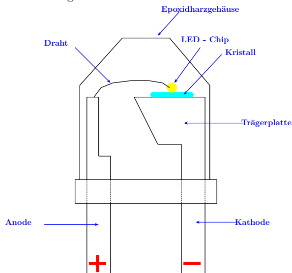
Figure 13.12.: Aufbau einer LED
