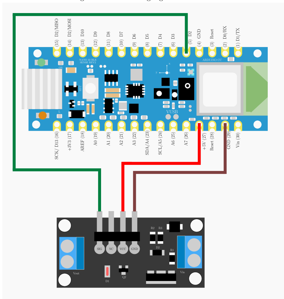
Figure 13.11.: Pinbelegung des MOS-FETs
