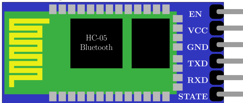
Figure 13.6.: Skizze des Bluetooth Moduls HC-05
