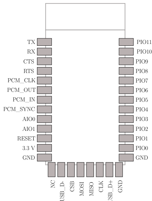
Figure 14.2.: Schnittstellen und Anschlüsse HC-05
