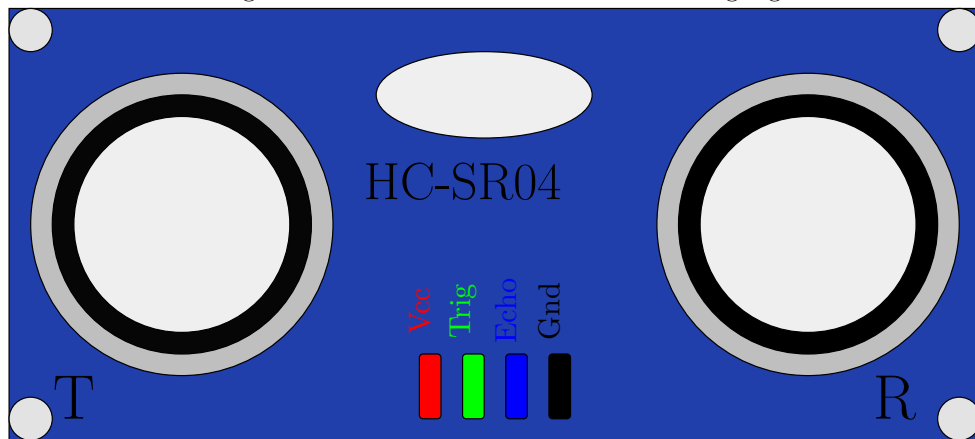
Figure 22.5.: Ultraschallsensor mit Pin-Belegung
