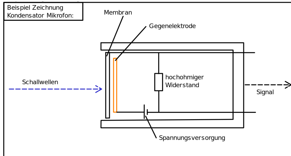
Figure 10.4.: Aufbau eines Kondensator Mikrofons
