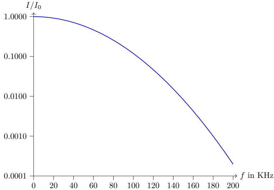
Figure 22.3.: Abnahme der Schallintensität in Abhängigkeit der Frequenz bei einem Meter, nach [HS23]
