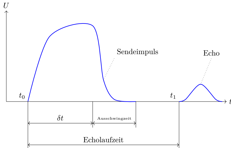
Figure 22.4.: Spannungsverlauf Schallwandler bei einer Echo-Laufzeit-Messung, nach [HS23]
