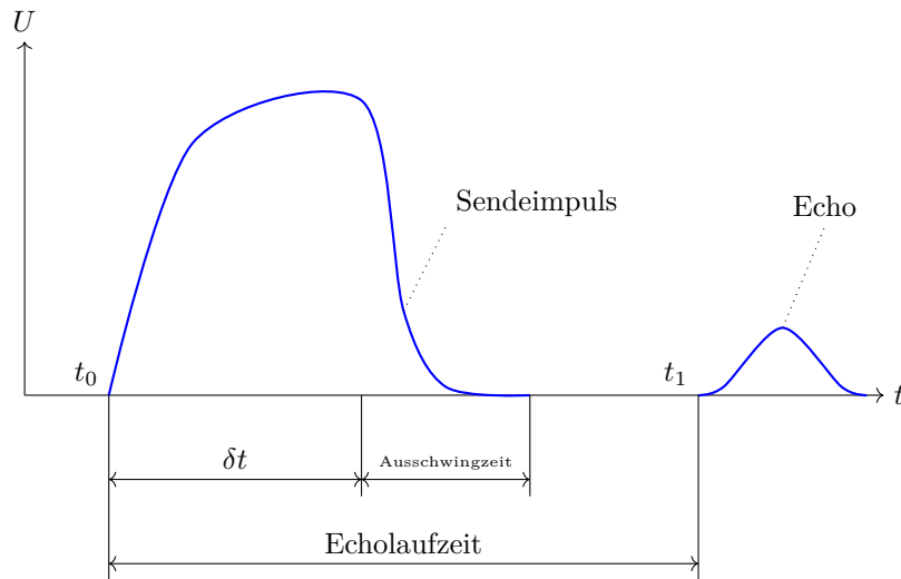
Figure 14.3.: Spannungsverlauf Schallwandler bei einer Echo-Laufzeit-Messung, nach [HS23]
