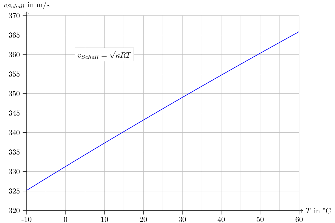
Figure 14.2.: Ausbreitungsgeschwindigkeit von Schall in Luft
