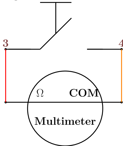
Figure 15.6.: Messen des Widerstands
