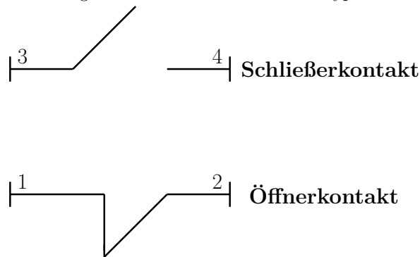
Figure 15.5.: Skizze der Schaltertypen
