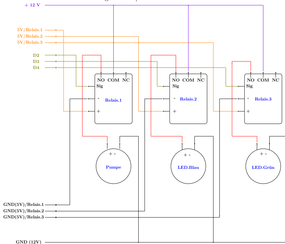
Abbildung 16.4.: 5/12 V Netz mit Aktoren
