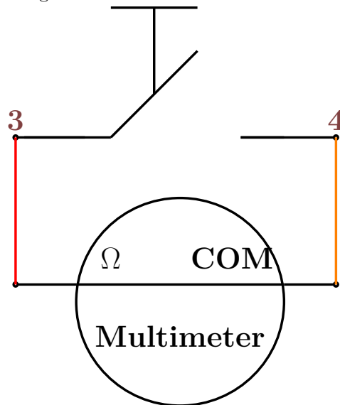
Figure 12.2.: Messen des Widerstands
