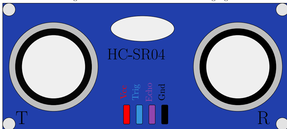
Figure 8.4.: Ultraschallsensor mit Pin-Belegung
