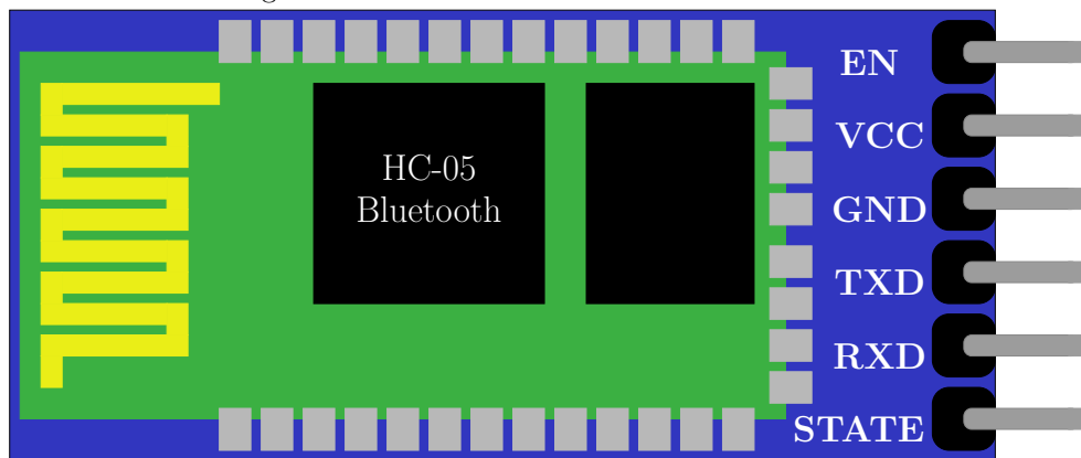
Figure 11.1.: Skizze des Bluetooth Moduls HC-05
