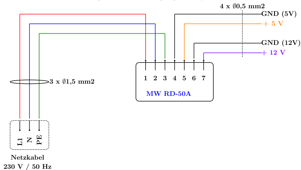
Figure 16.2.: Versorgungsschaltplan
