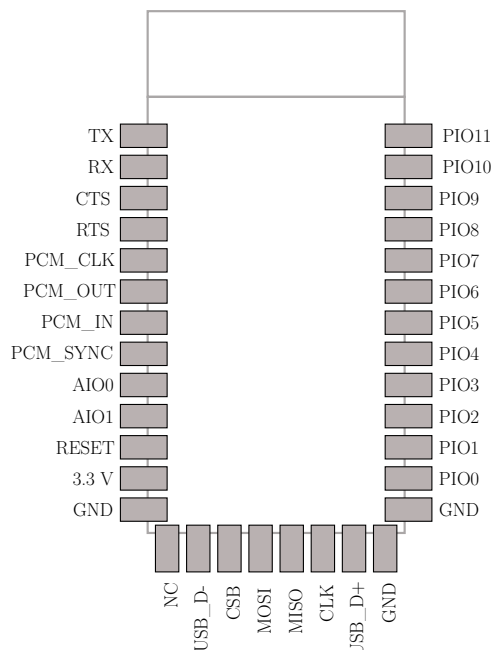
Figure 11.2.: Schnittstellen und Anschlüsse HC-05
