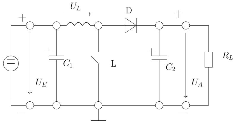
Figure 5.2.: Aufwärtswandler
