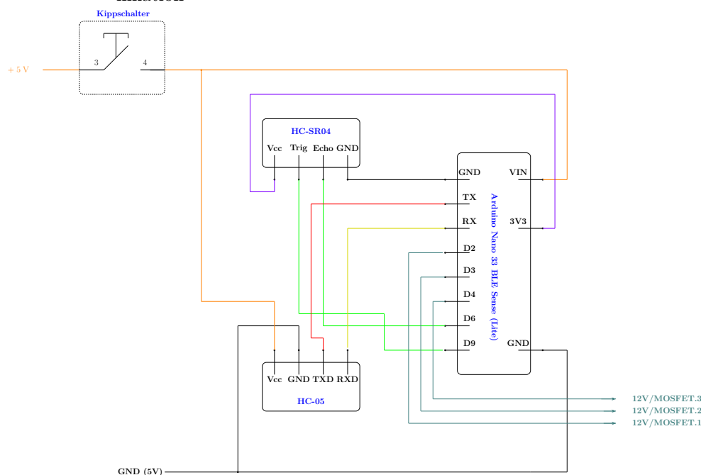
Figure 16.3.: Schaltplan: Arduino-basierte Steuerungseinheit mit Bluetooth-Kommunikation
