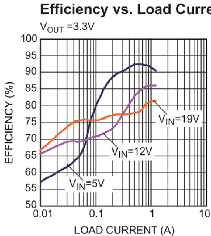
Figure 5.7.: Spannungswandler Wirkungsgrad [MPS15]
