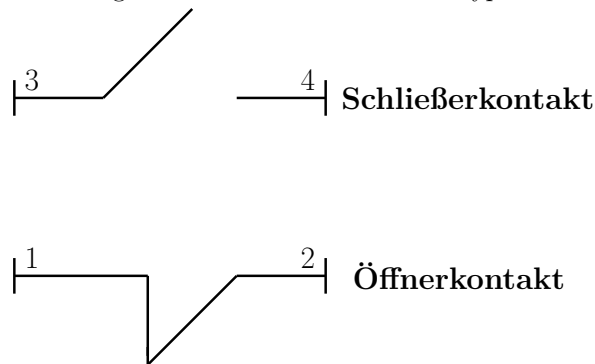
Figure 13.7.: Skizze der Schaltertypen
