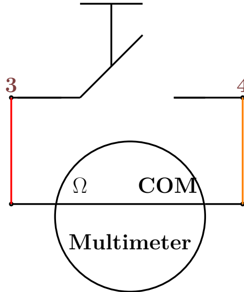
Figure 13.8.: Messen des Widerstands
