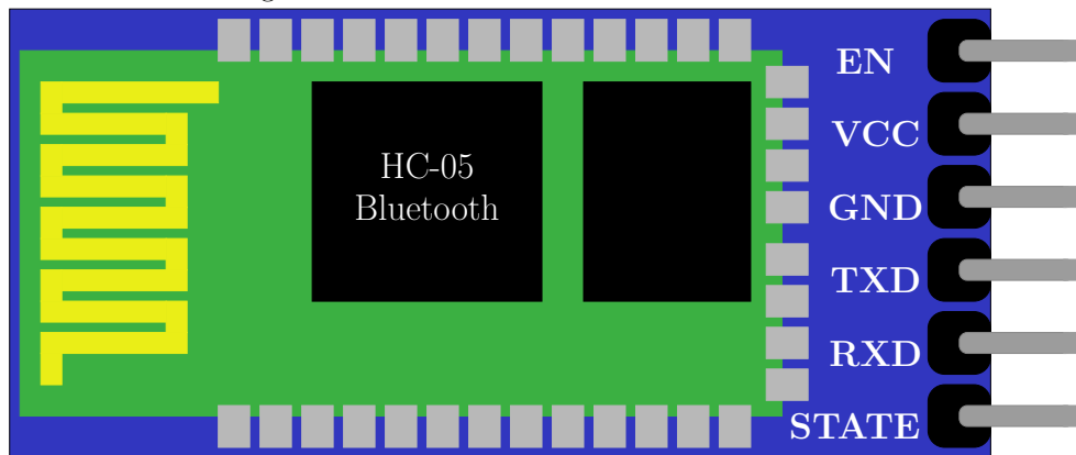
Figure 13.6.: Skizze des Bluetooth Moduls HC-05
