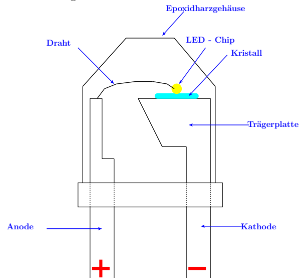
Figure 13.11.: Aufbau einer LED
