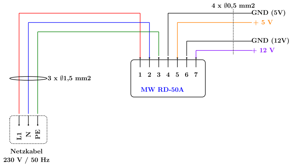
Abbildung 16.2.: Versorgungsschaltplan
