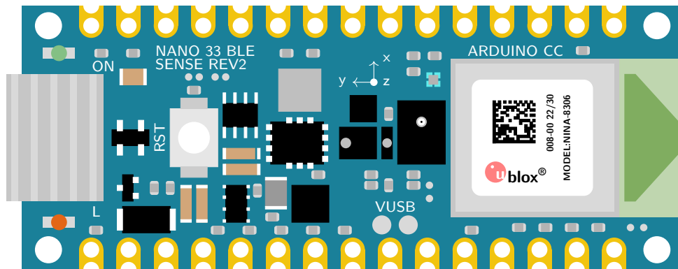
Abbildung 4.1.: Arduino Nano 33 BLE Sense Rev. 2, siehe Arduino Store
