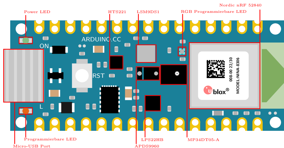
Abbildung 4.4.: Anordnung der Sensoren auf dem Board
