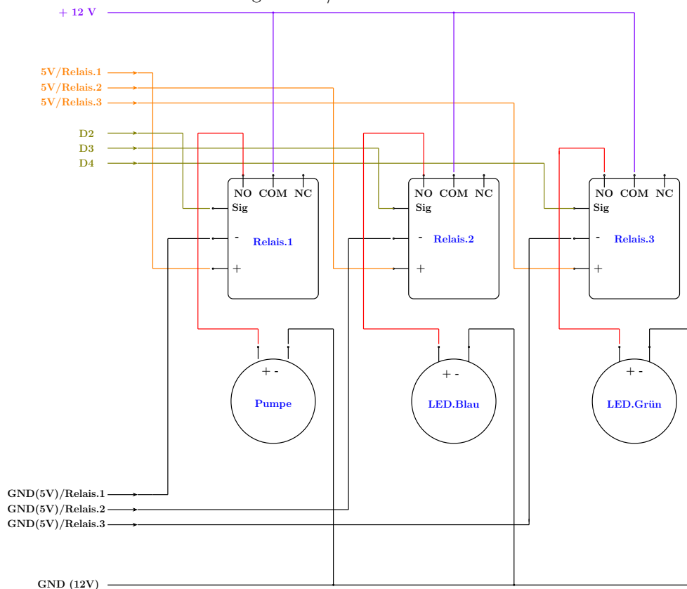
Abbildung 17.4.: 5/12 V Netz mit Aktoren
