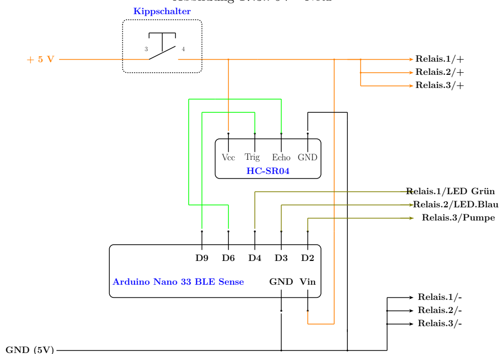
Abbildung 17.3.: 5V - Netz
