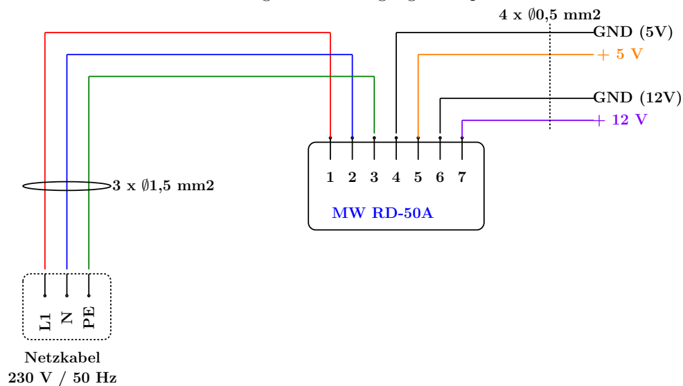
Abbildung 17.2.: Versorgungsschaltplan
