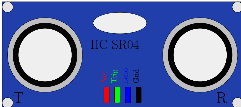
Figure 27.4.: Ultraschallsensor mit Pin-Belegung
