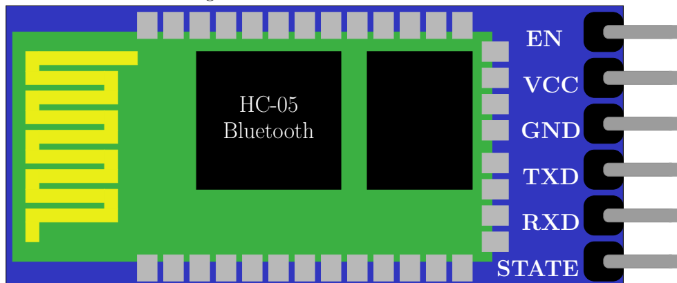
Abbildung 10.1.: Skizze des Bluetooth Moduls HC-05
