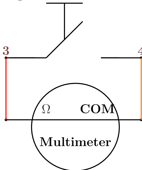
Figure 9.2.: Messen des Widerstands
