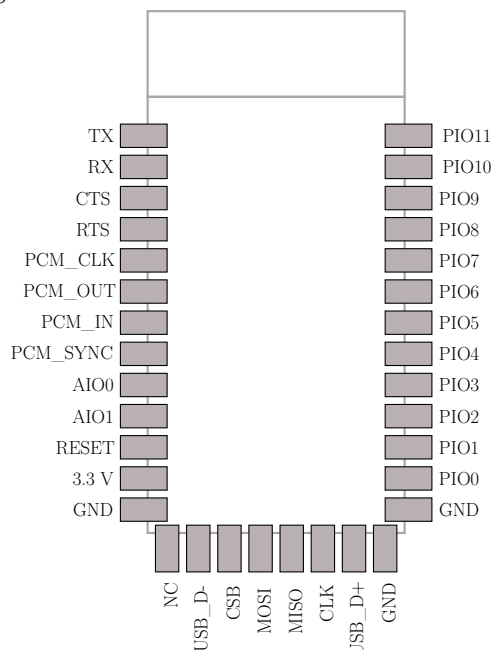
Figure 8.2.: Schnittstellen und Anschlüsse HC-05
