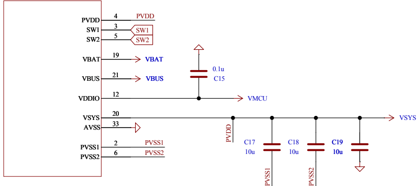
U4B NPM1300-QEAA-R7
