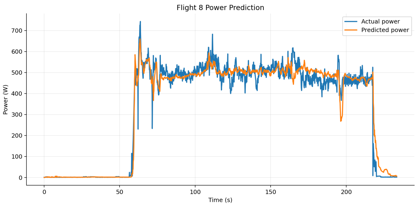
flight 8 功率时序
