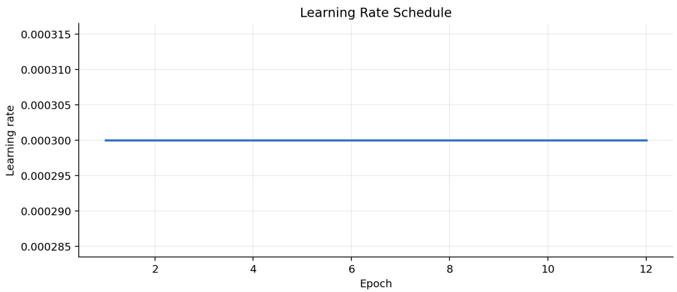
学习率变化
