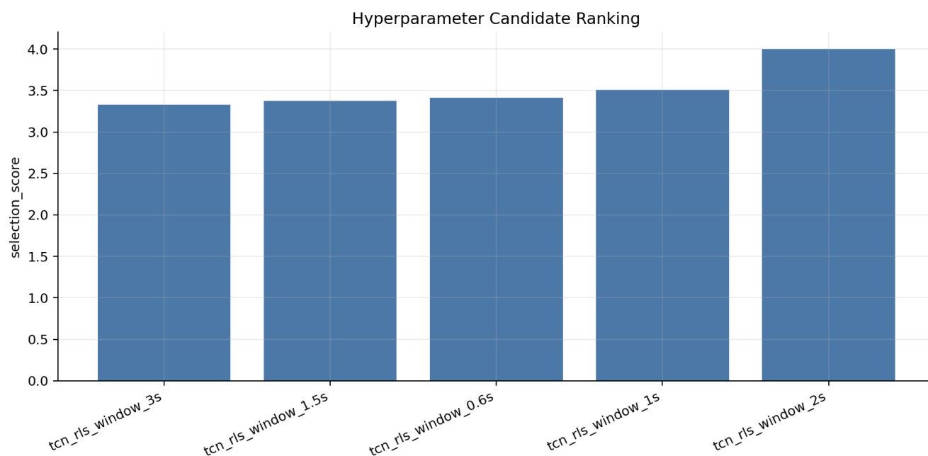
超参数排序
