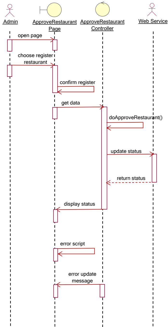
รูปที่ 3.143 ซีเควนซ์ไดอะแกรมระดับ 1 ของยูสเคส Approve Restaurant
