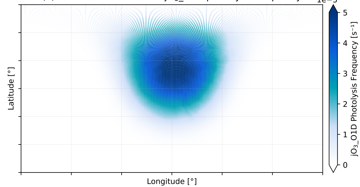
(d) 2024-07-02 00:00 UTC jO 3 _O1D photolysis frequency
