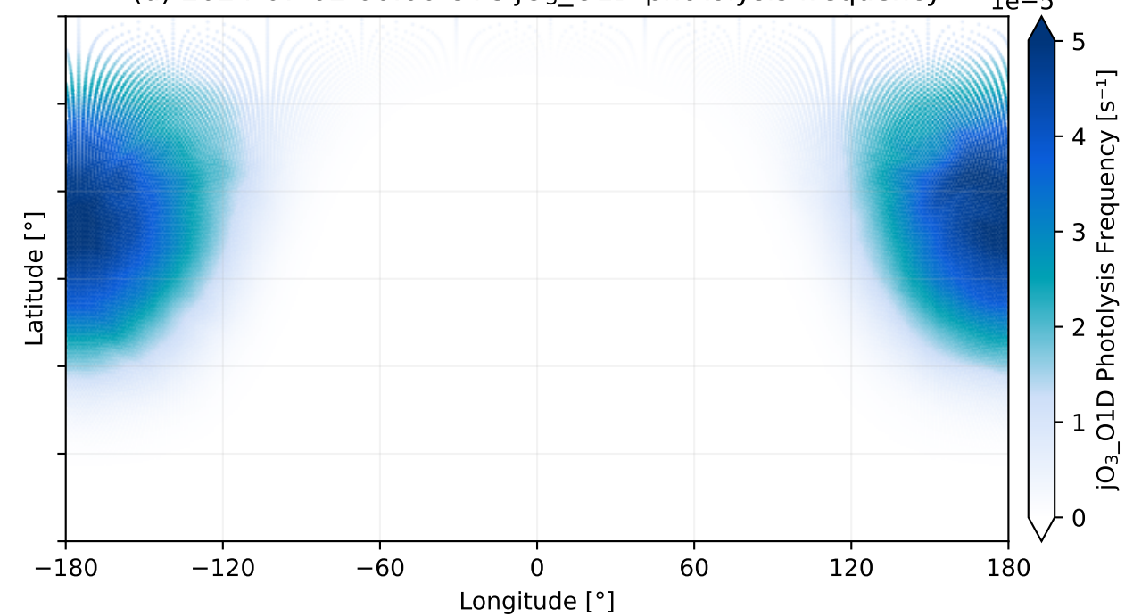
(d) 2024-07-02 00:00 UTC jO 3 _O1D photolysis frequency
