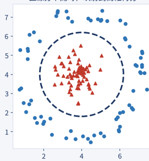
③ 核技巧 Kernel 直線分不開時，映射到高維再分
