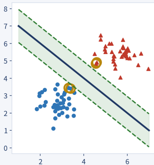
② SVM：選間隔最寬的那條 圈起來的是「支持向量」
