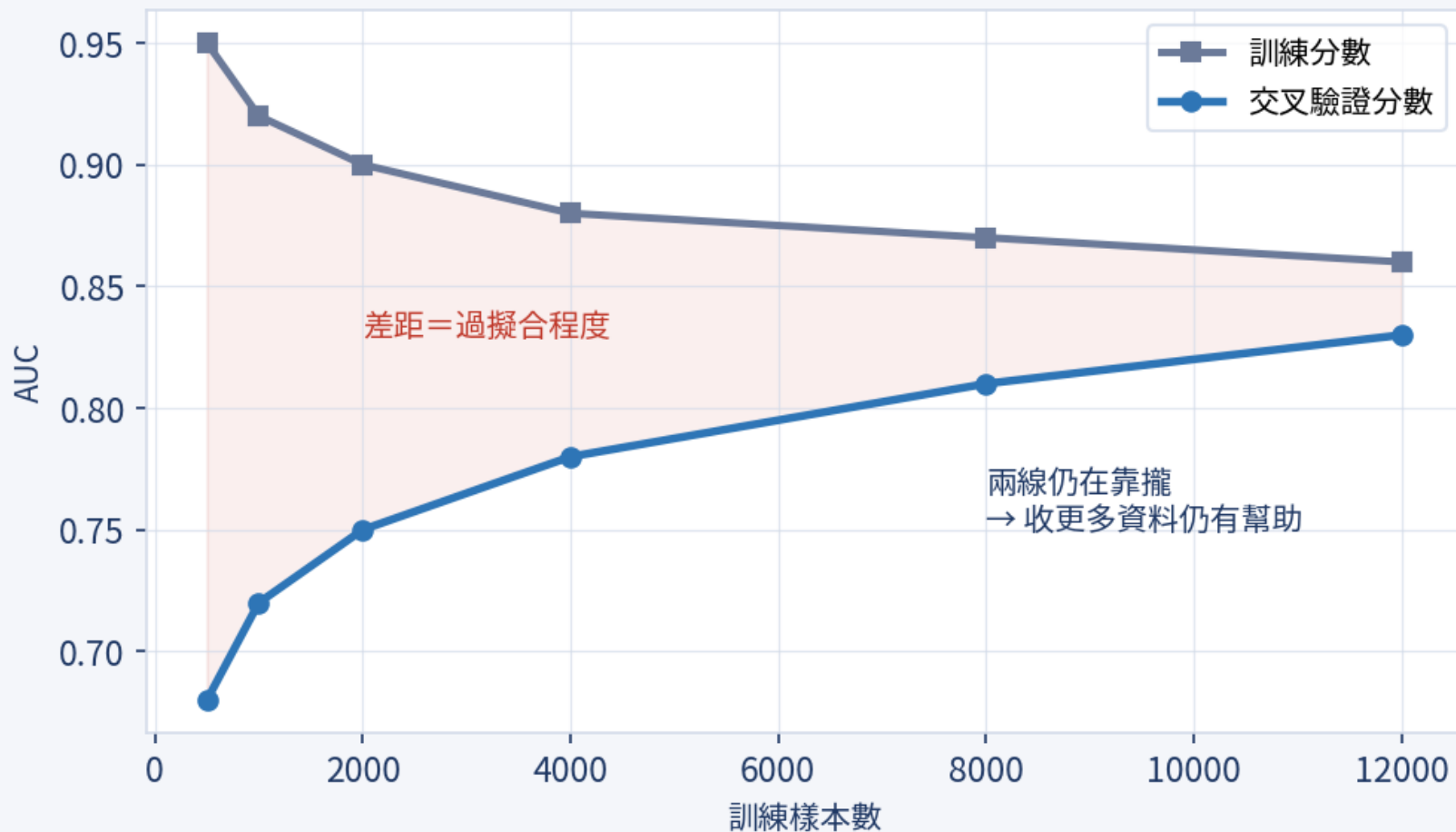
學習曲線：資料夠了嗎？
