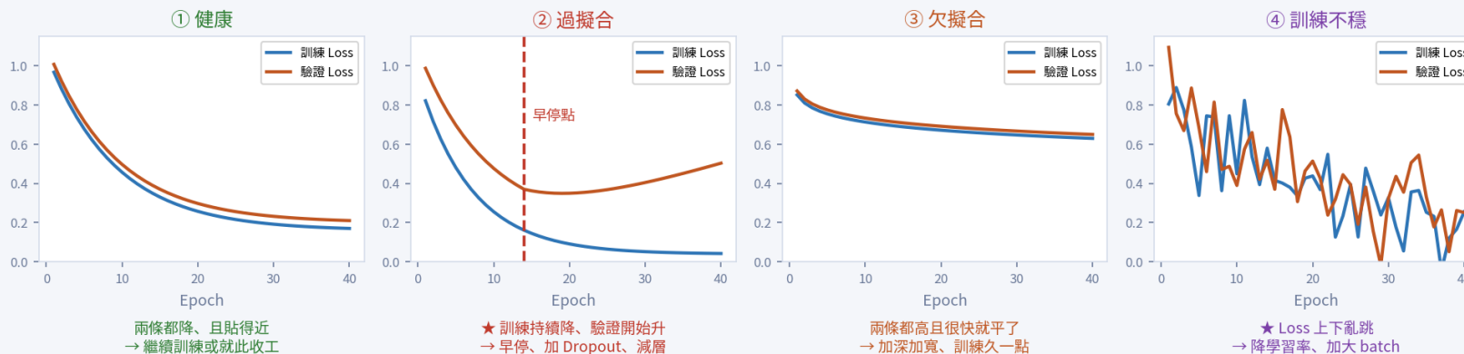
讀懂 Loss 曲線：四種樣態與各自的處方
