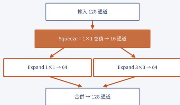
SqueezeNet : Fire Module
