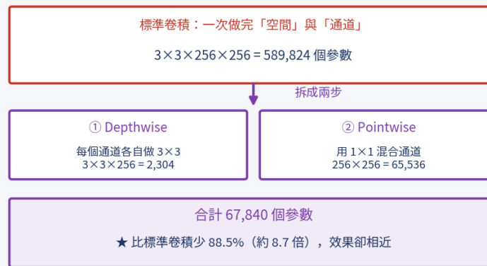
Xception : 深度可分離卷積
