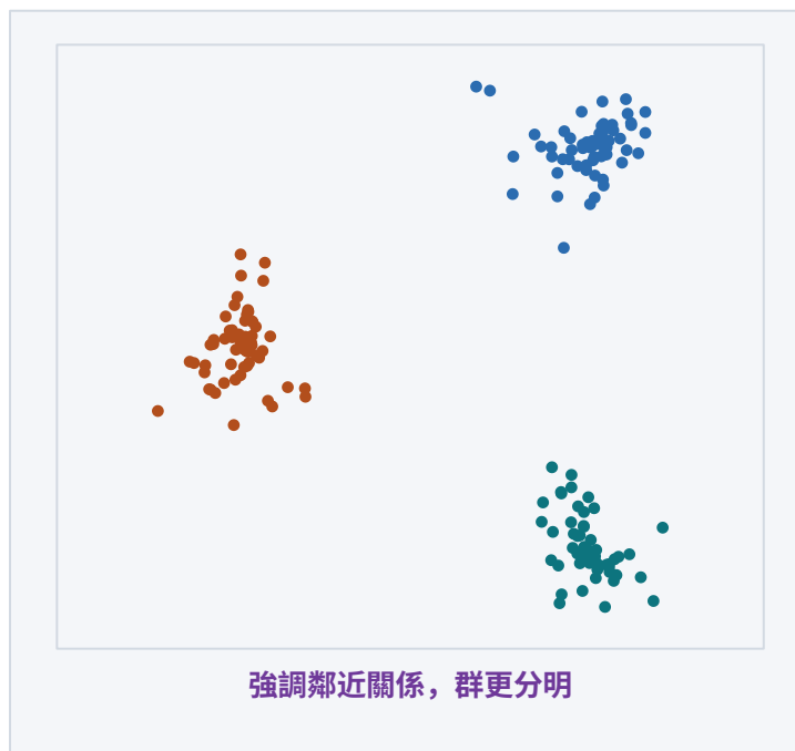
右・t-SNE：非線性
