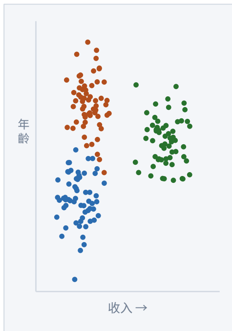
左・真實結構
