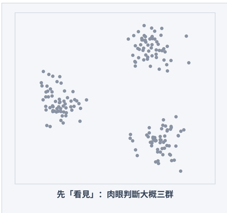
左・先 PCA 降到 2 維（還沒分群）
