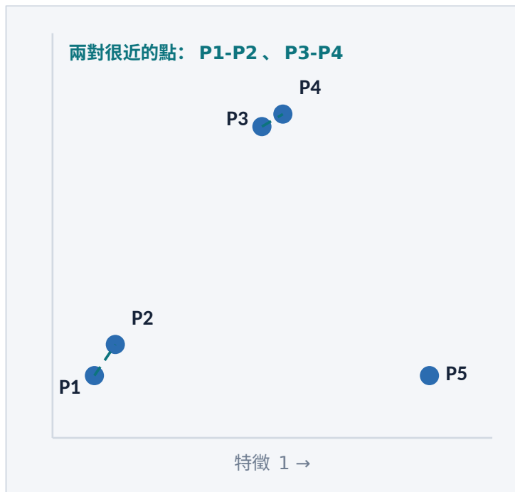
左・五個資料點
