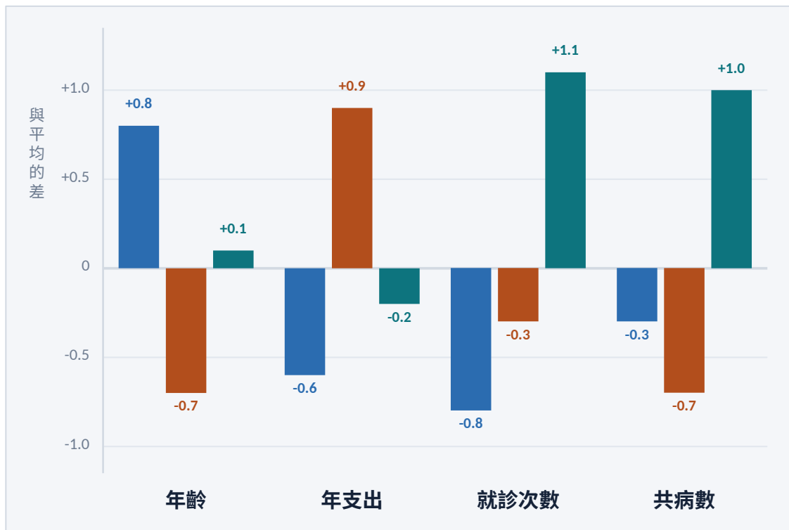
各群在四個特徵上與整體平均的差（標準化後）
