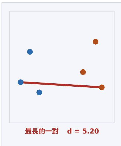
中・完全連結 Complete
