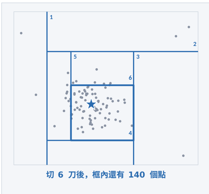
左・正常點：密集區
