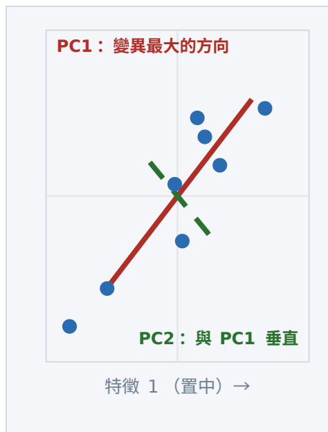
② 置中後找主成分方向
