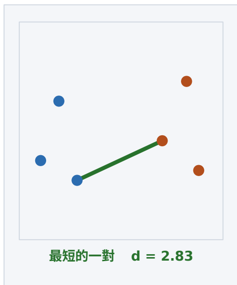
左・單一連結 Single
