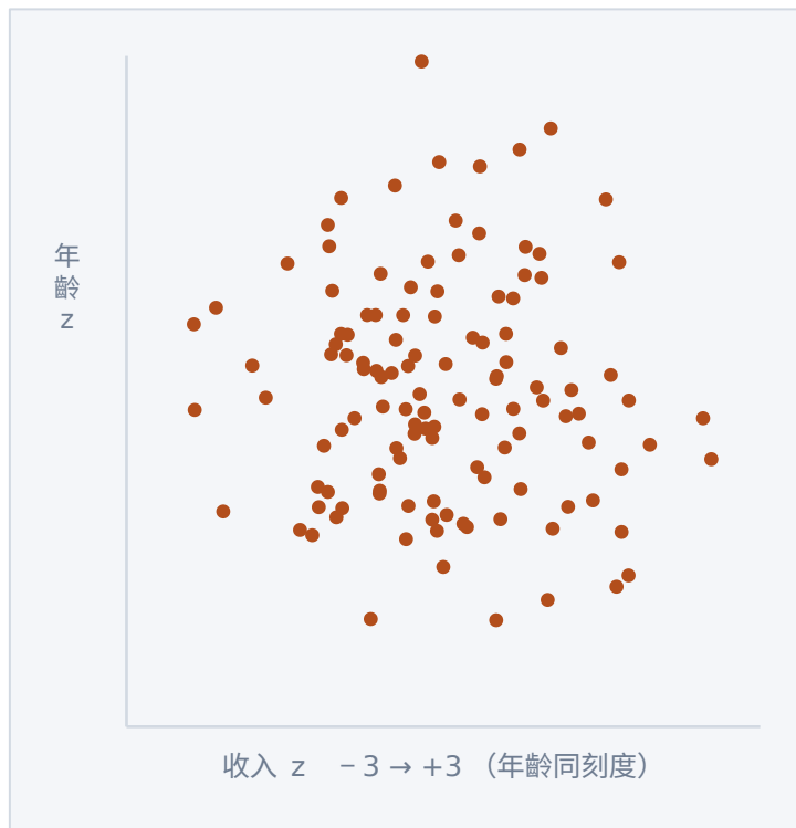
右・Z-Score 標準化後
