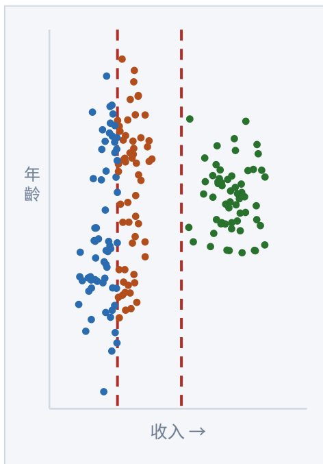
中・未正規化 (純度 77%)
