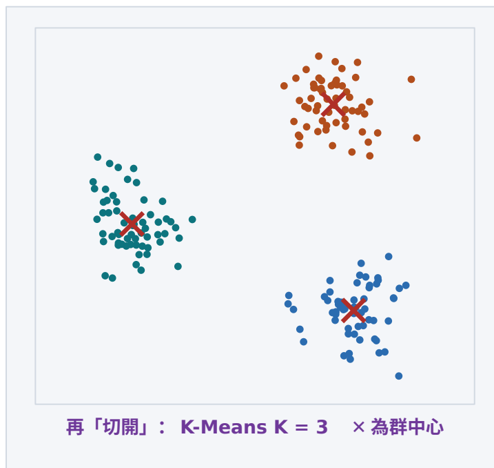
右・在原始空間分群，用同一張圖上色
