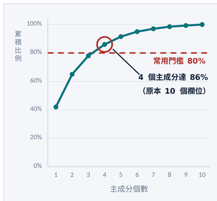
右・累積解釋變異
