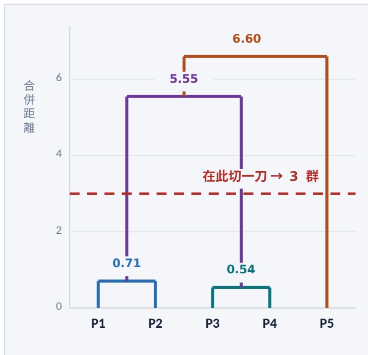
右・樹狀圖 Dendrogram
