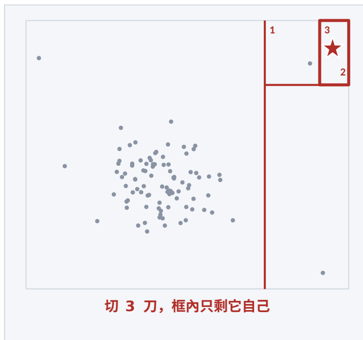
右・異常點：稀疏區
