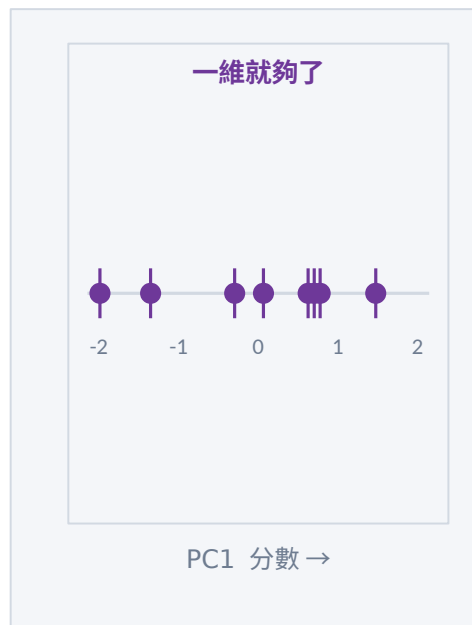
③ 投影到 PC1（1 維）
