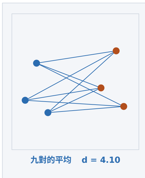
右・平均連結 Average
