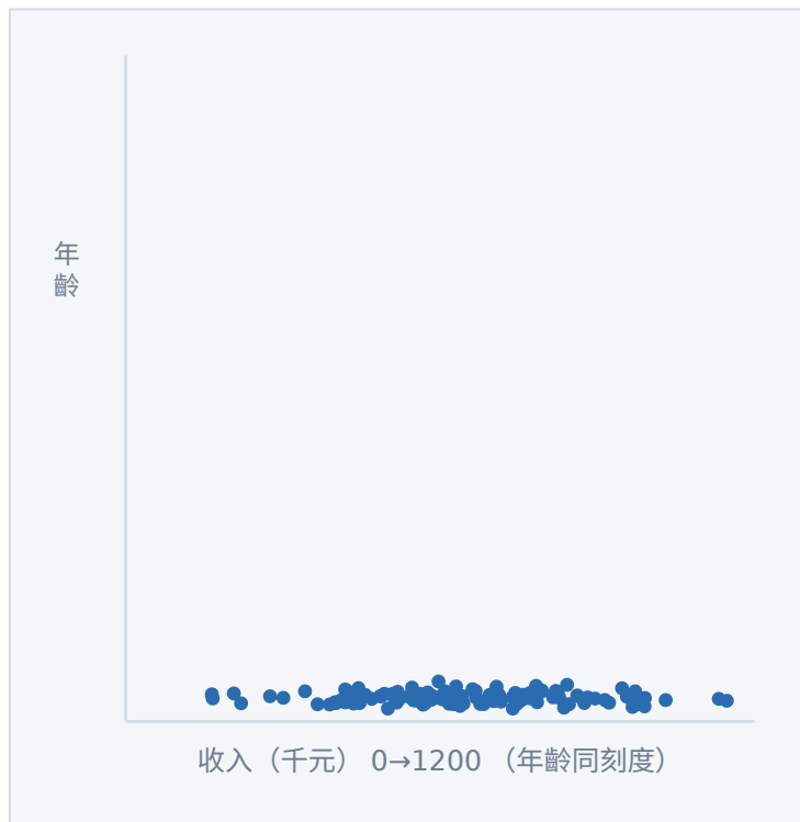
左・原始尺度（兩軸同刻度）
