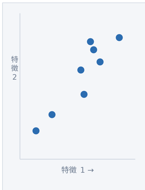
① 原始資料（2 維）
