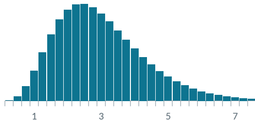
樣本平均的分佈（每次抽 n = 5 ）
