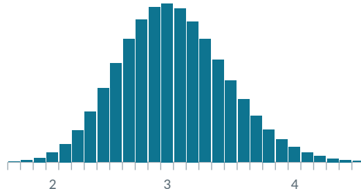
樣本平均的分佈（每次抽 n = 50 ）
