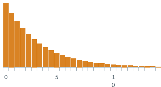
母體（明顯右偏，平均 3）
