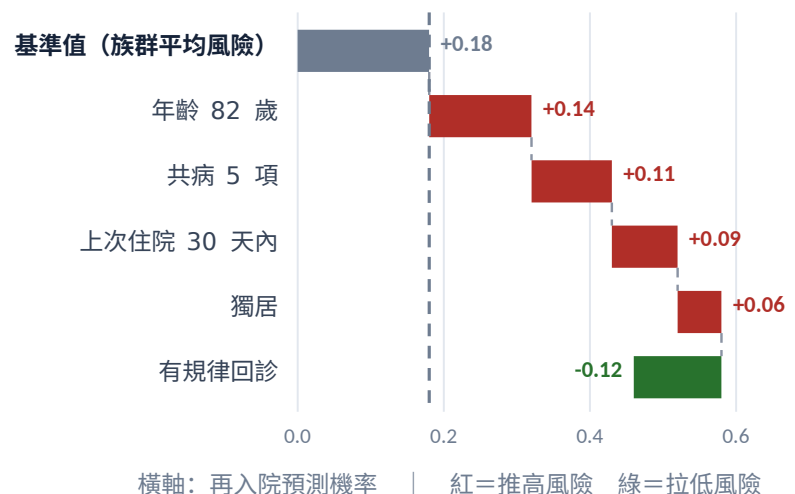
SHAP 瀑布圖：這一位病人為什麼被判高風險
