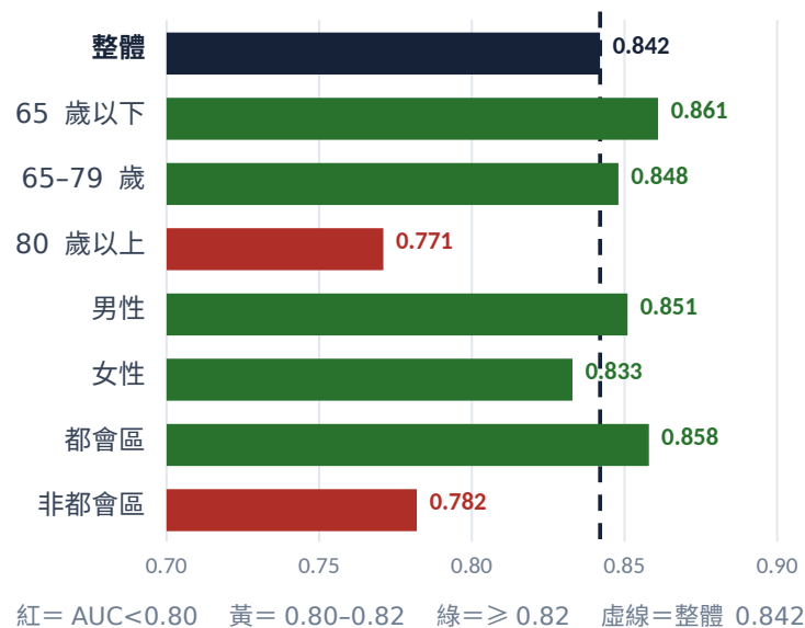
同一個模型，拆到子群體去看 AUC
