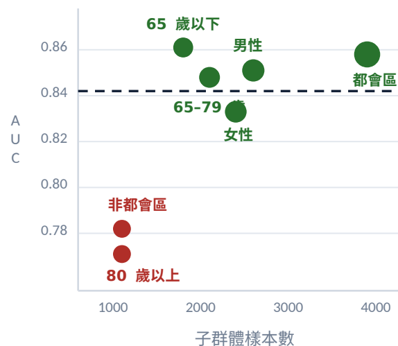
樣本數少的群體，表現往往也差
