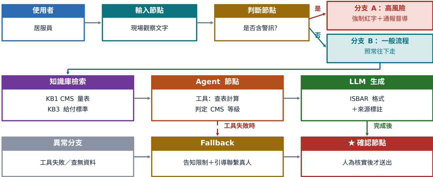
長照 CMS 評估與通報 Agent：六樣東西都要在圖上看得到
