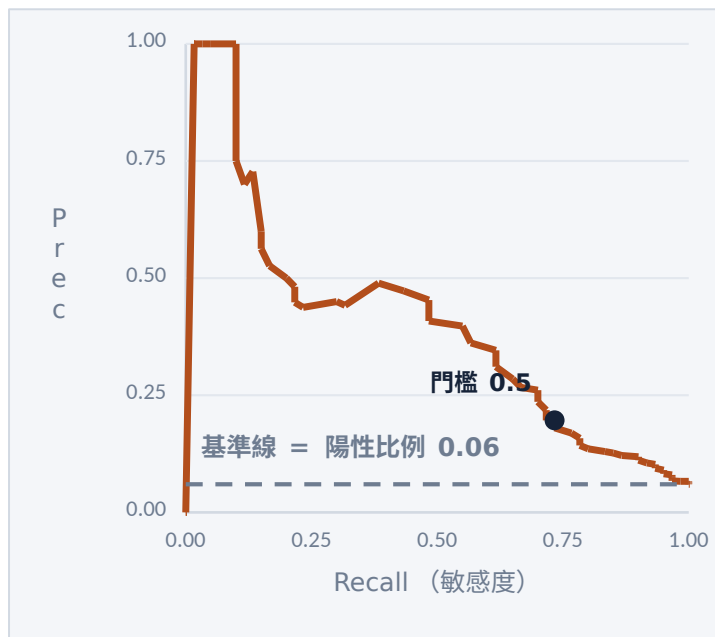
右・PR 不平衡資料更誠實
