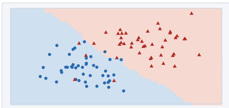
③ k-NN (k=15)：貼著資料的曲線
