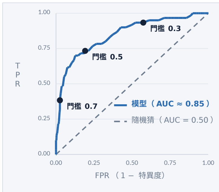
左・ROC 每個門檻是曲線上一點
