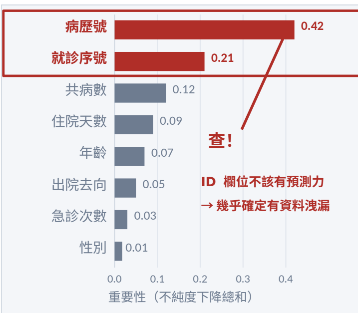
右・紅色警訊：ID 類欄位排最前面
