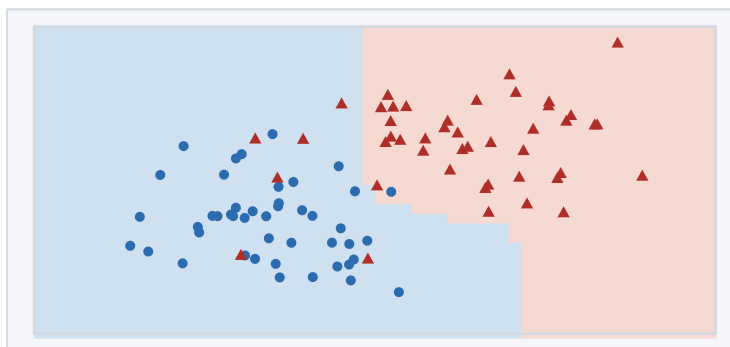
④ 隨機森林：平滑化的階梯
