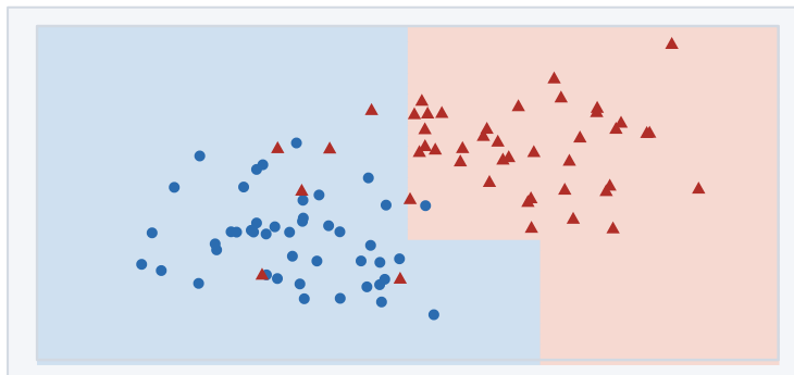
② 決策樹：軸平行的階梯
