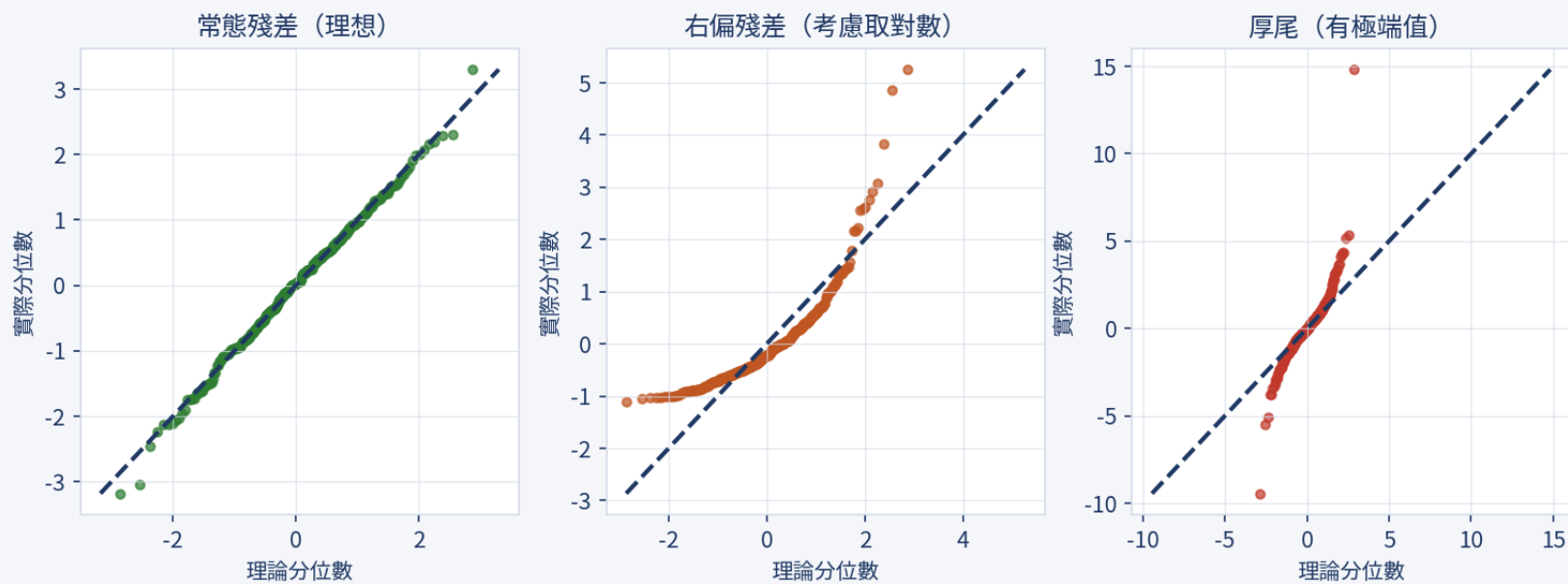
Q-Q 圖：點貼著對角線 = 殘差接近常態
