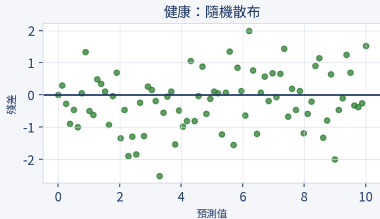
殘差圖四種型態：先看形狀，再看 R^2
