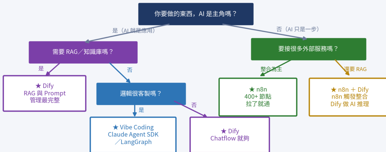
選型決策樹：這個需求該用哪個工具？
