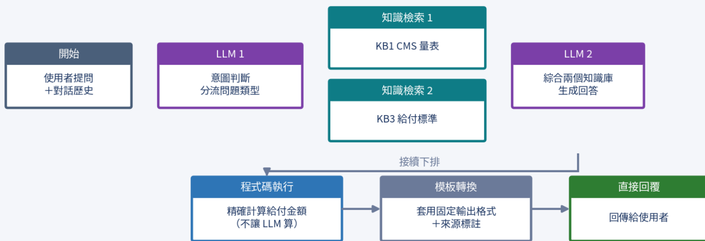
模式三 Chatflow：對話 + 條件分支
