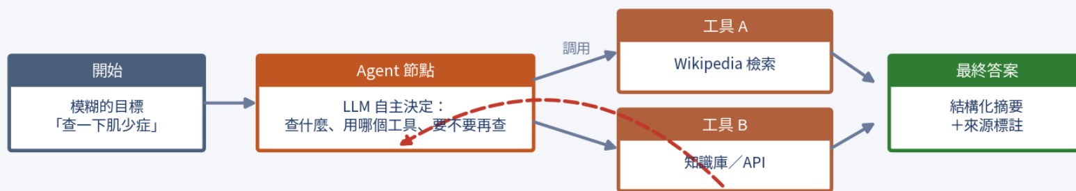
模式四 Agent : LLM 自己決定下一步
