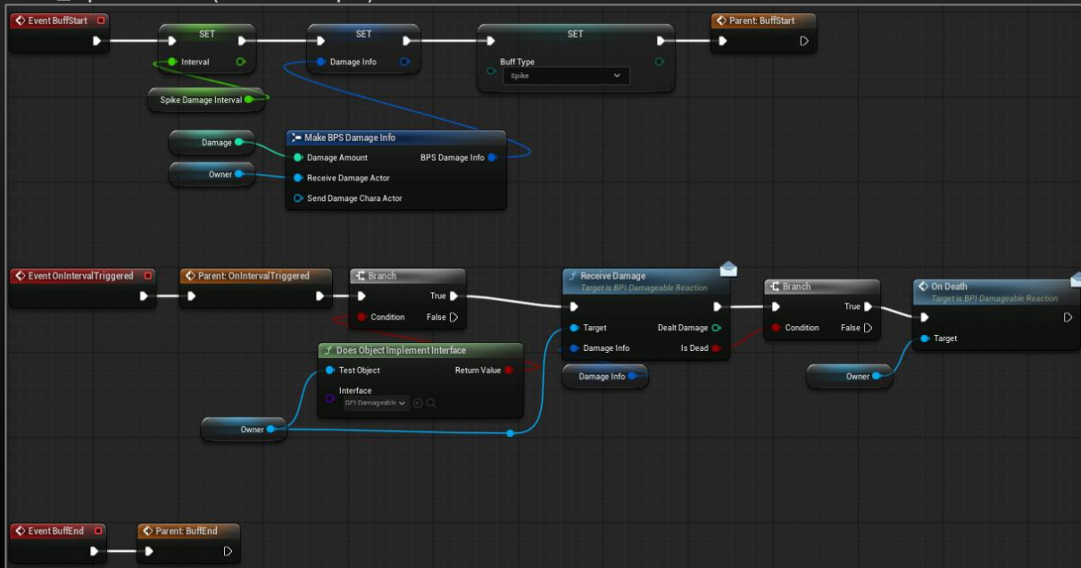
BP_SpikeEffect(Event Graph)
