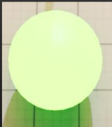
BP_Grapple
