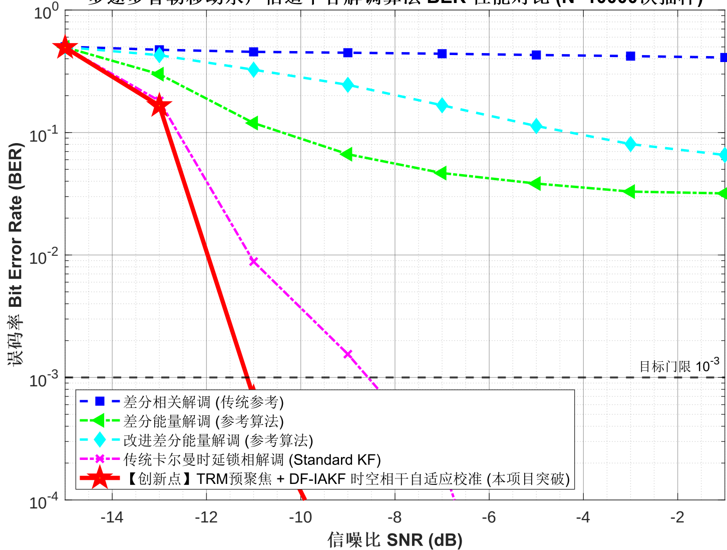
多途多普勒移动水声信道下各解调算法 BER 性能对比 (N=10000次抽样)
