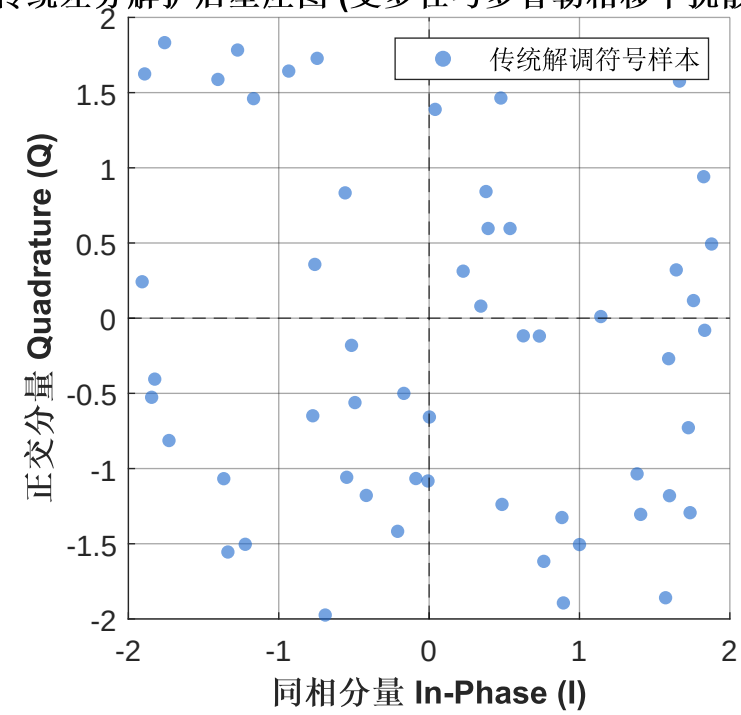
传统差分扩后星座图 (受多径与多普勒相移干扰严重) 【创新点】 TRM+DF-IAKF 自适应相漂校准后星座图 (清晰)
