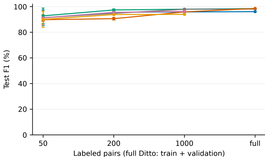
DBLP-ACM
