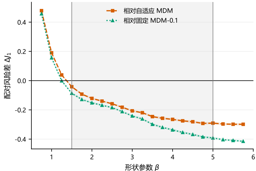
B 直接估计相对结构路线的风险差
