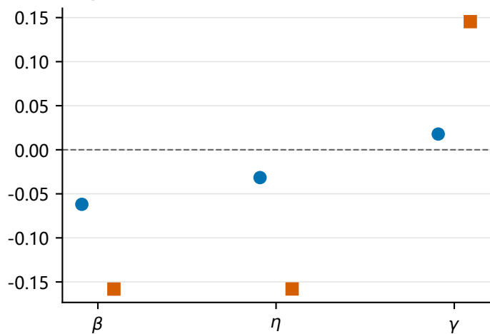
B 标准化 Bias
