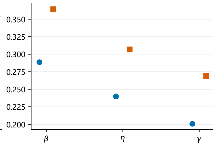
D 标准化 RMSE
