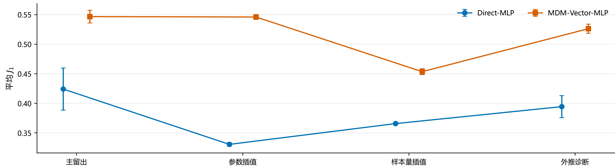
B 标准化 Bias
