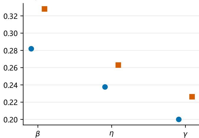
C 标准化 SD
