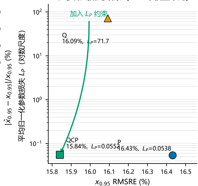
C 广参数域配对结果 (200 个模型单元)
