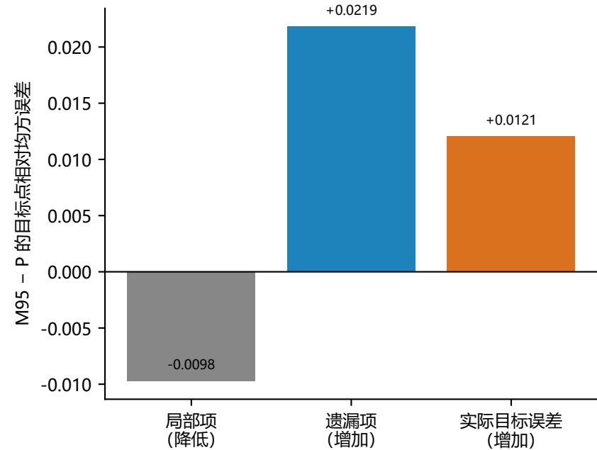
C 遗漏项反转局部近似的改善
