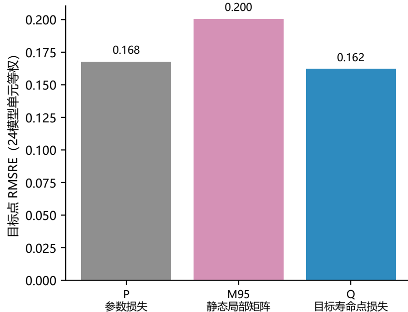
B 静态代理未复现 Q 的精度
