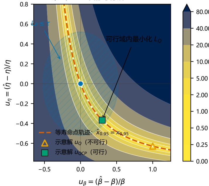
B 约束 L_P \leq \tau 下的可行解
