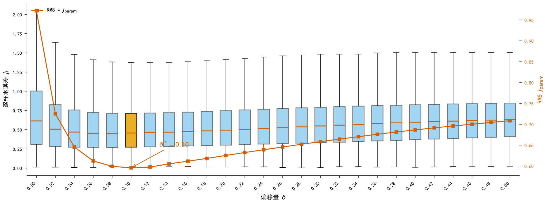
固定 \delta 下逐样本误差 j_i 的分布 (27配置 \times 500rep, 共13,500样本/ \delta )
