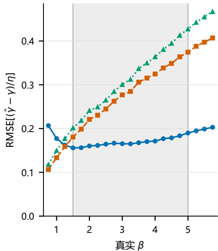
C 位置参数
