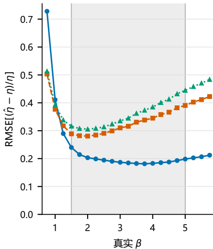
B 尺度参数
