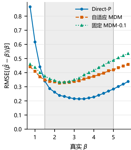
A 形状参数
