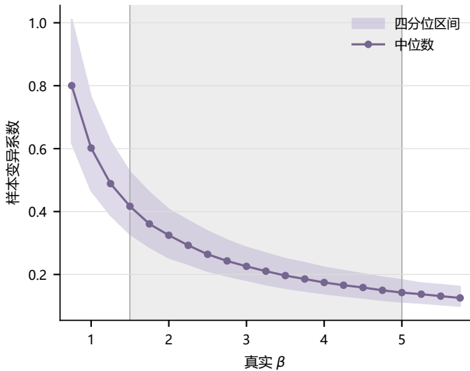
A 样本变异系数
