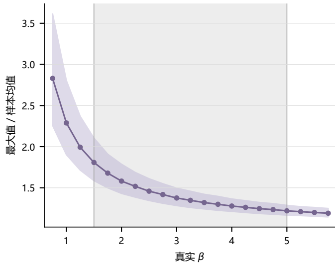
B 最大值 / 样本均值
