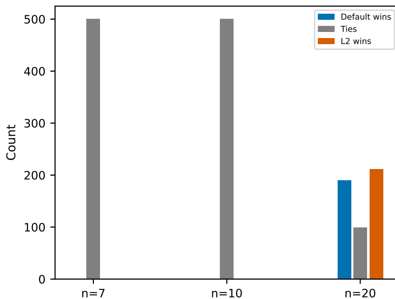
Default vs L2 Paired
