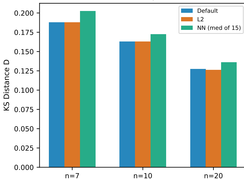
Default vs L2 Paired
