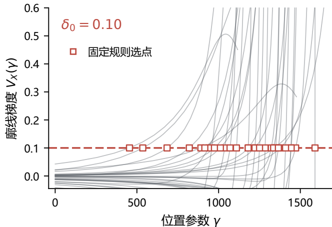
a 固定偏移 MDM
