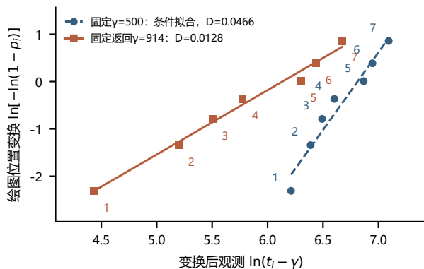
d 原 \beta=5, n=7 , 组#11: 七个样本点与条件回归直线
