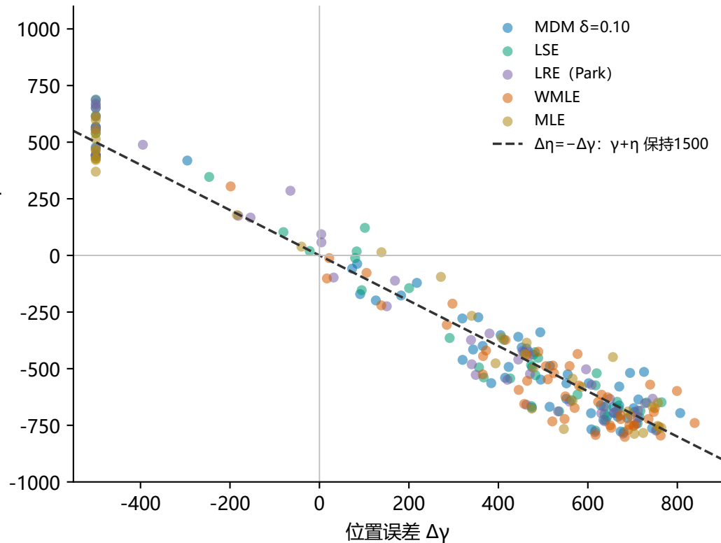
同组估计沿“位置增、尺度减”方向补偿
