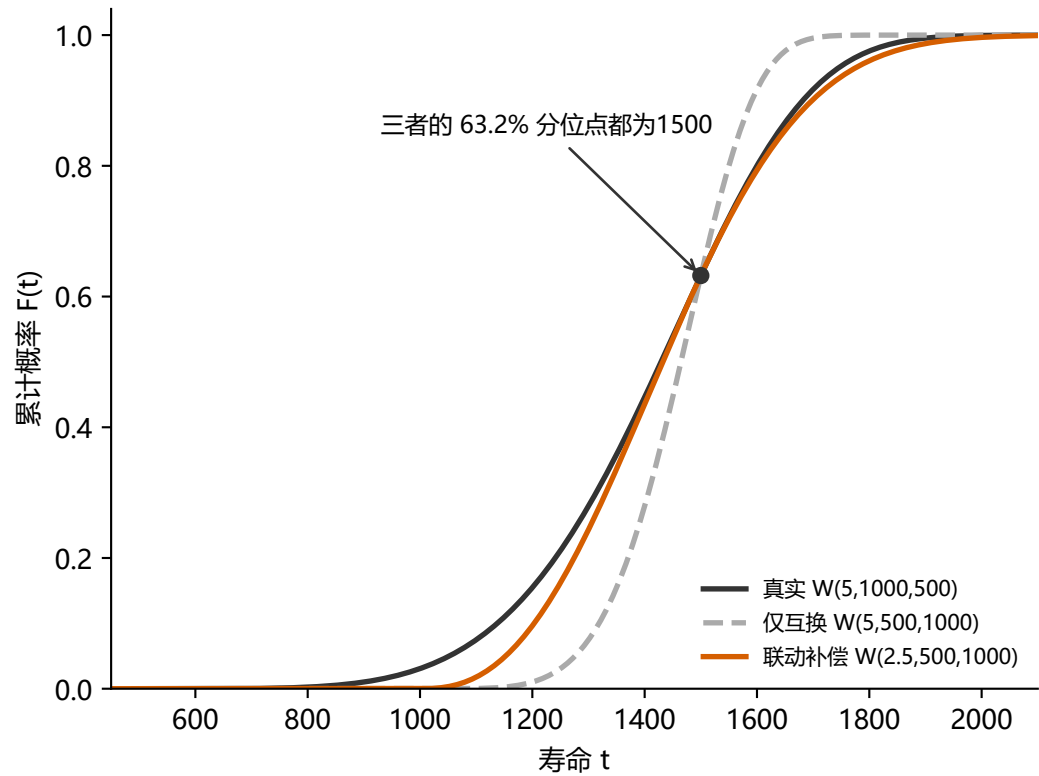
形状同步改变后，分布中部更接近真实
