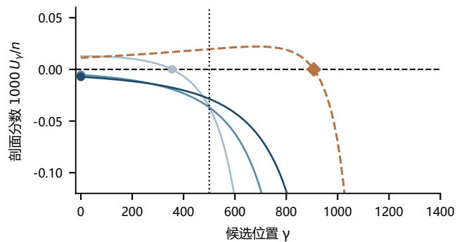
d MLE: 有限极大或 \gamma=0 边界
