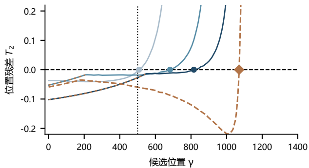
c WMLE: 位置方程的零点
