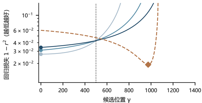
c WMLE: 位置方程的零点
