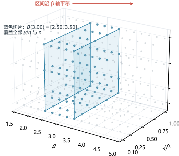
a 参数空间中的 \beta 区间
