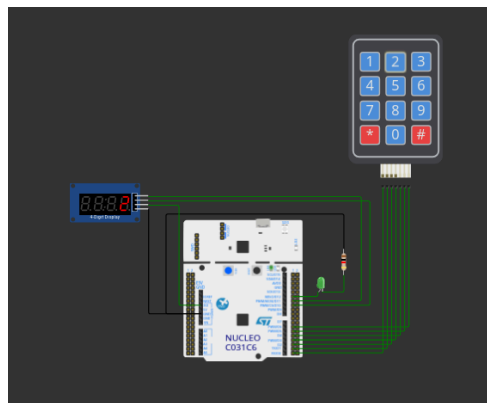
Рис. 4. На клавиатуре было введено число 2 - второй операнд
