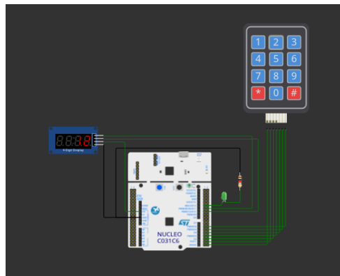
Рис. 2. На клавиатуре было введено число 12 - первый операнд
