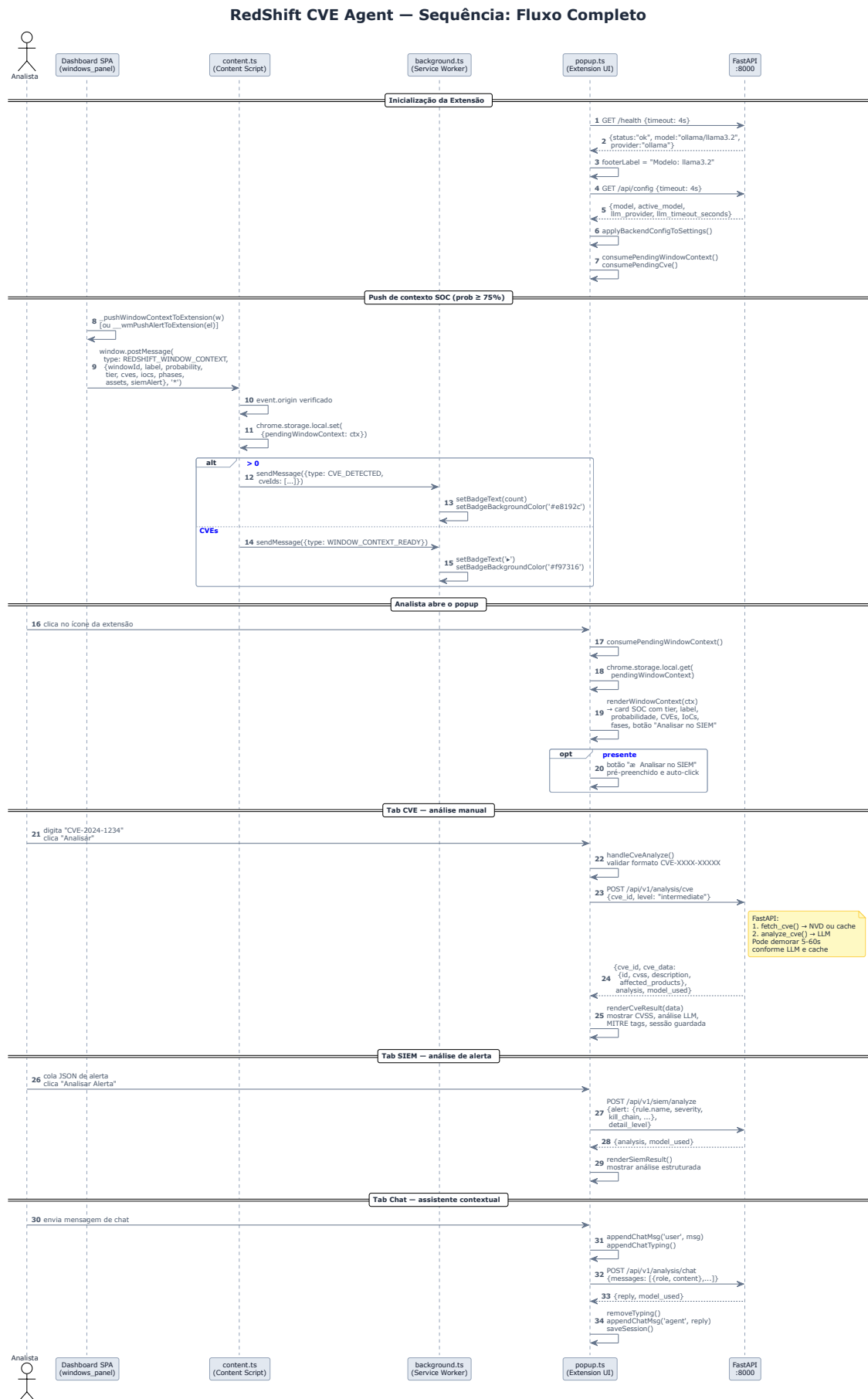
Figure 1: Sequência: Fluxo Completo
