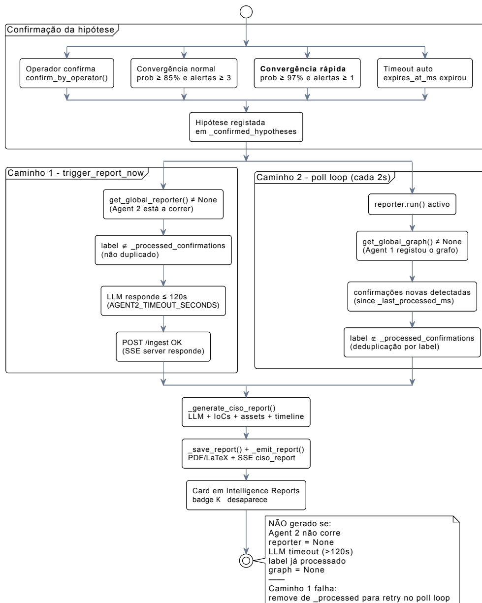
Figure 4: Condições para a geração de Relatórios
