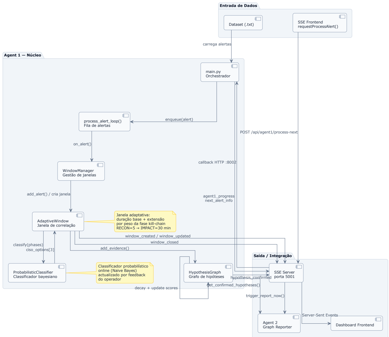
Figure 1: Arquitetura de Componentes
