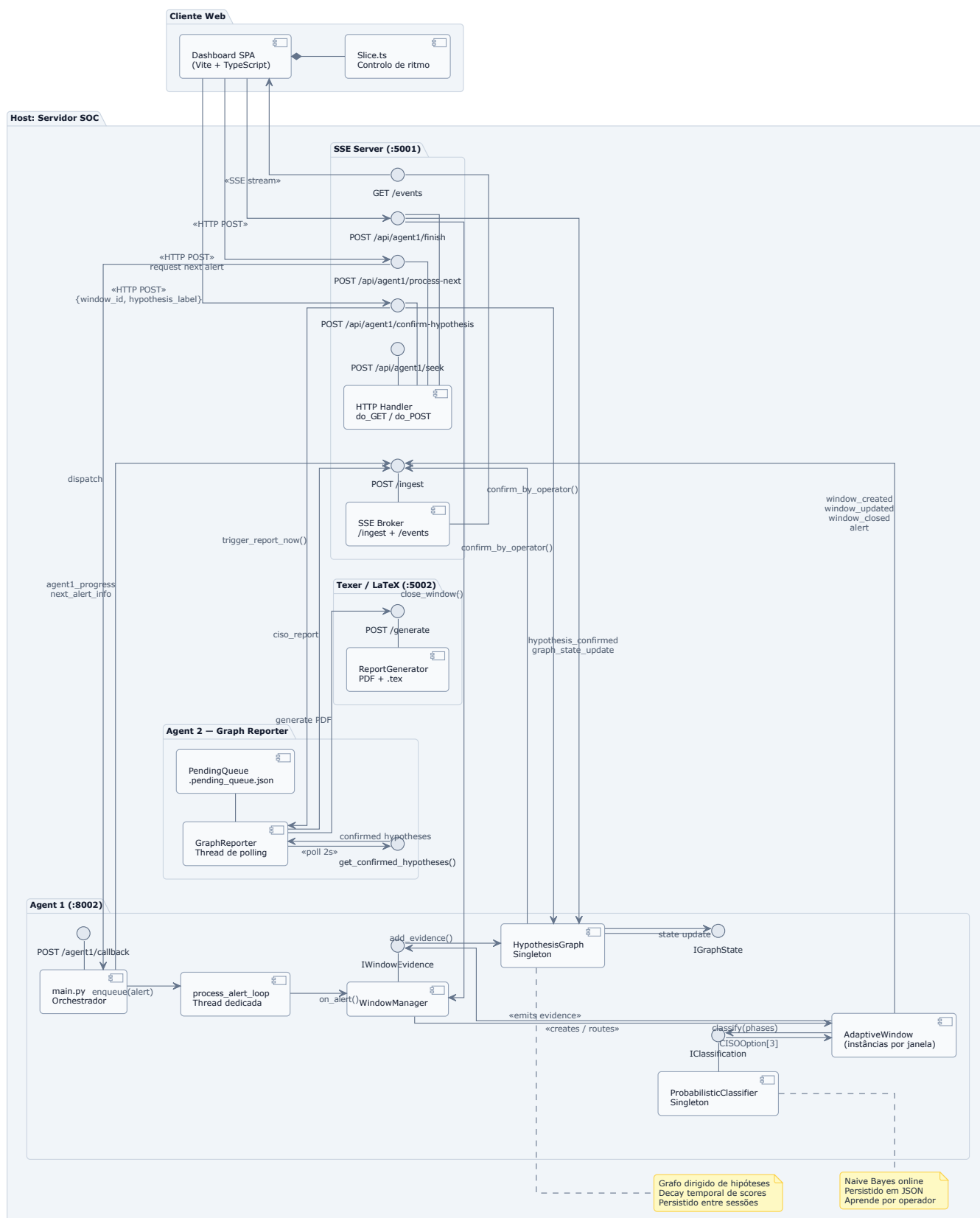
Figure 2: Diagrama de Componentes e Interfaces
