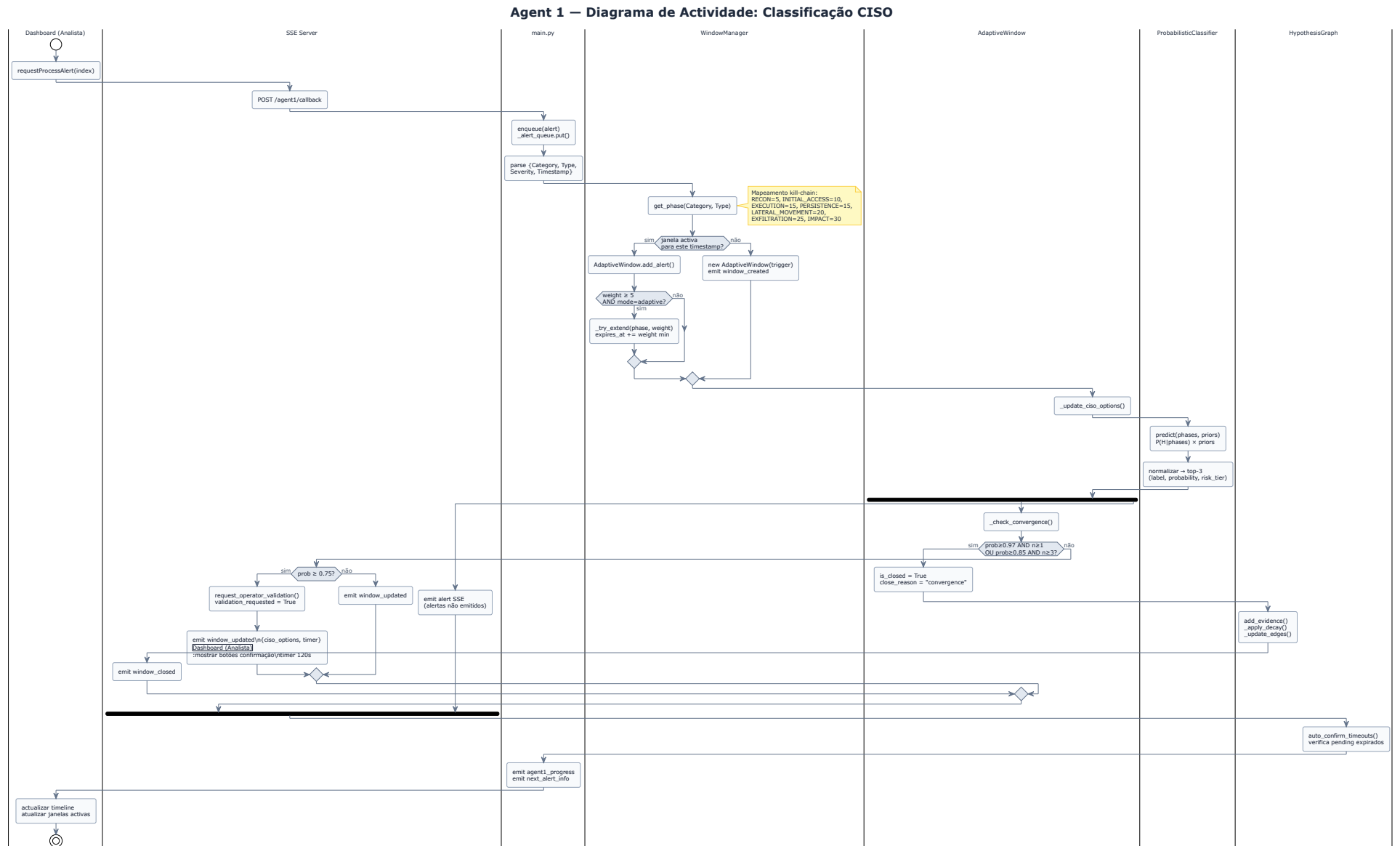
Figure 5: Diagrama de Actividade: Classificação CISO
