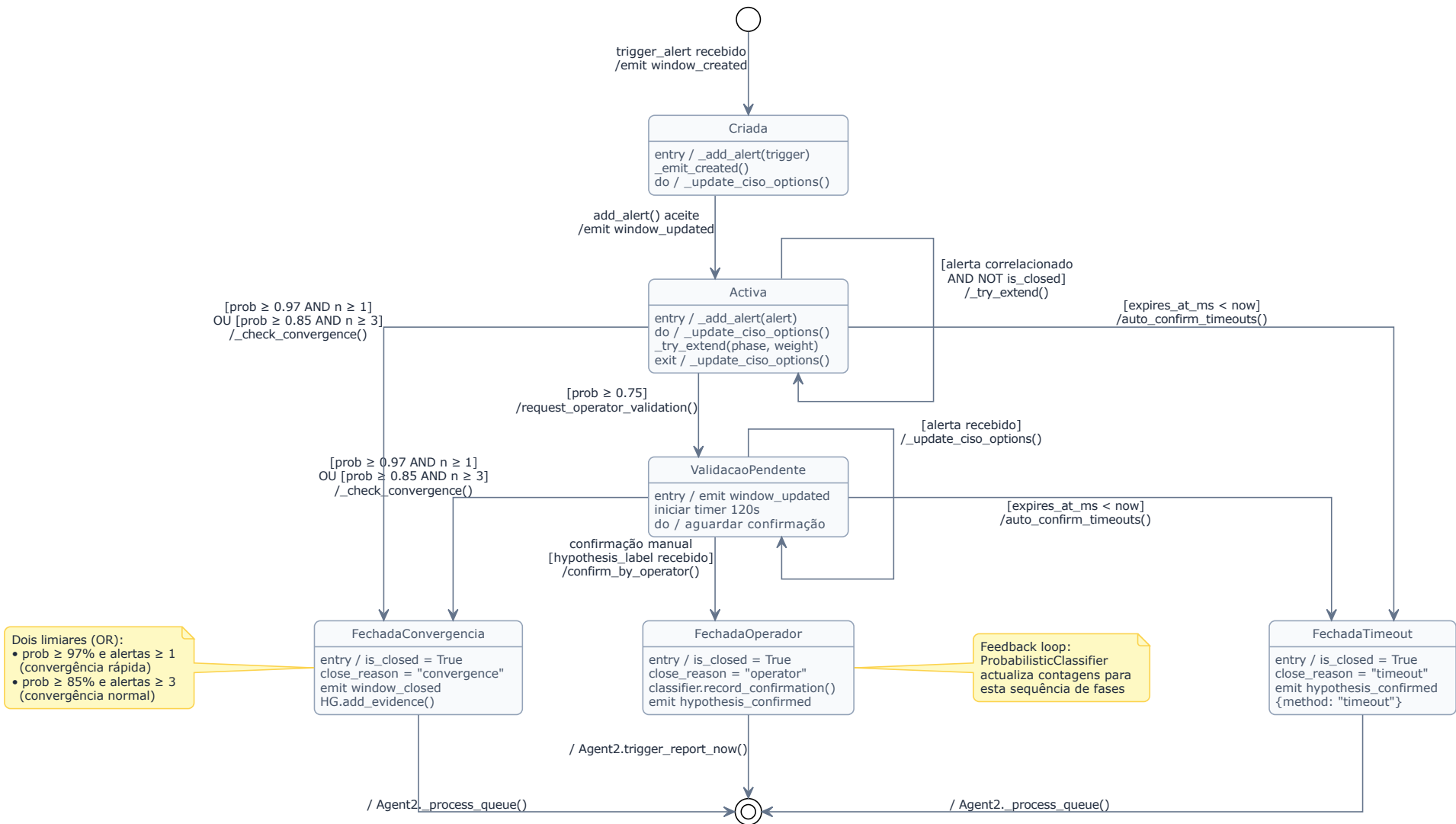
Figure 4: Máquina de Estados: AdaptiveWindow
