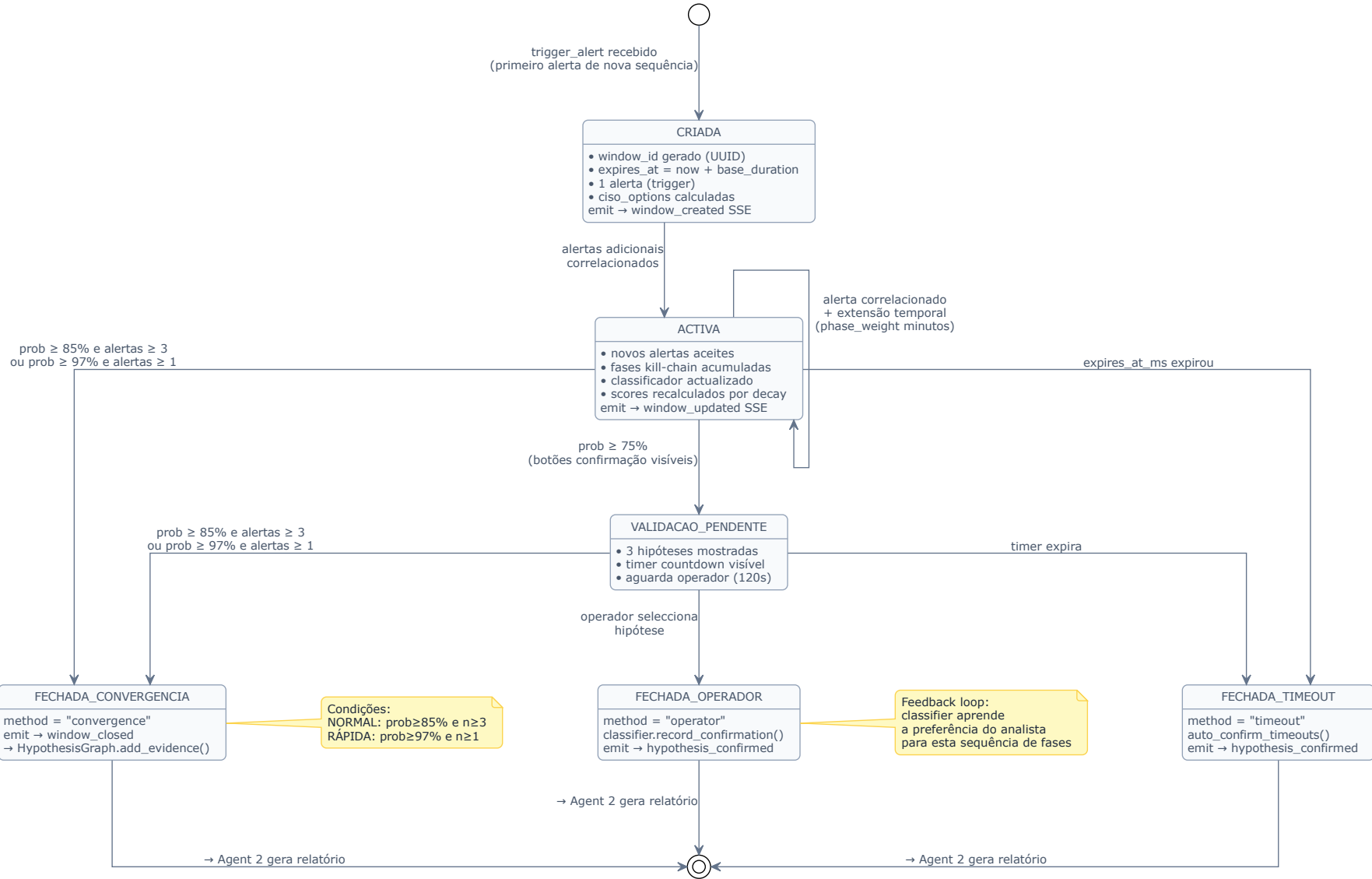
Figure 2: Ciclo de Vida da Janela Temporal
